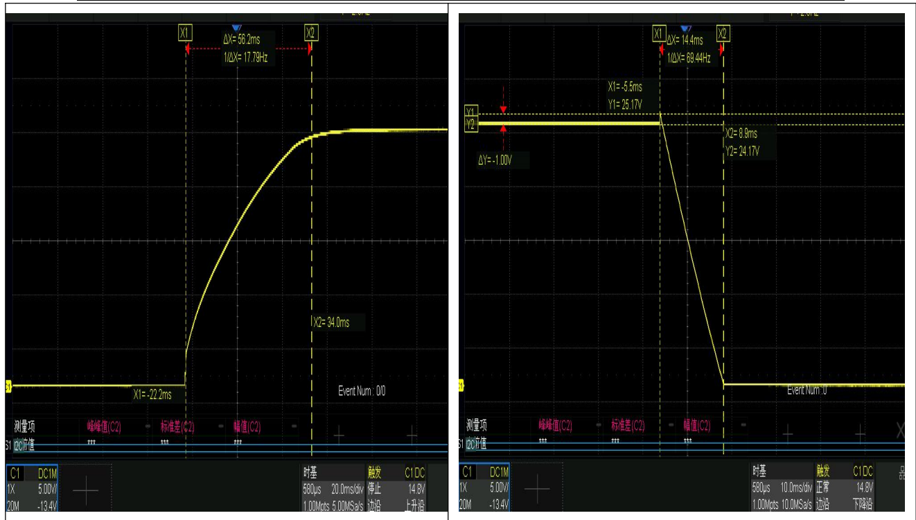
图(5) 25% ~ 50%负载动态波形
